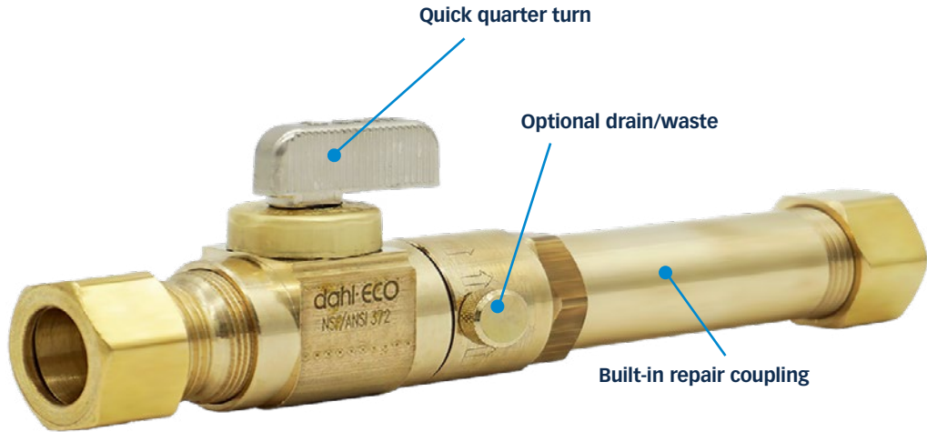
#521LB-33-33LD 5/8 OD Comp x 5/8 OD Comp Long with Drain/Waste
